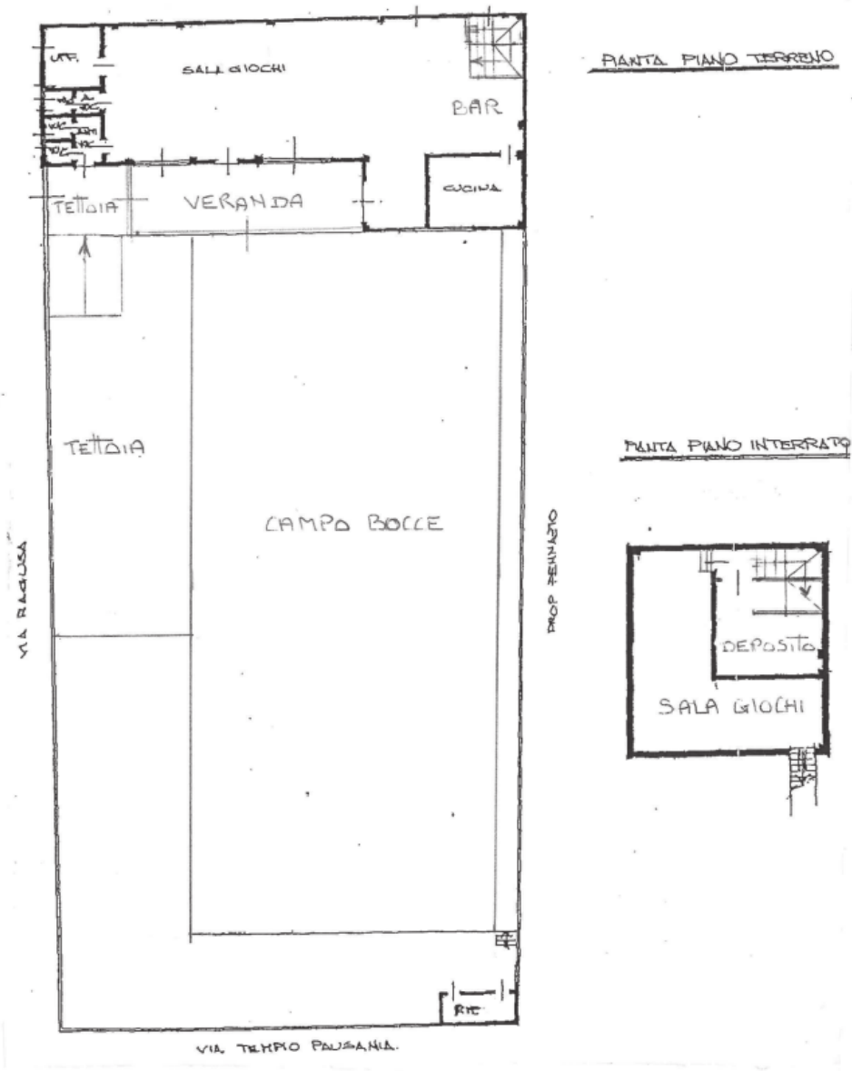
Pianta piano terreno. Foglio 1392 Particella 75 subalterno 1
